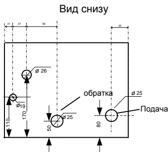
Рисунок 3 Профиль панели трубопроводов.
